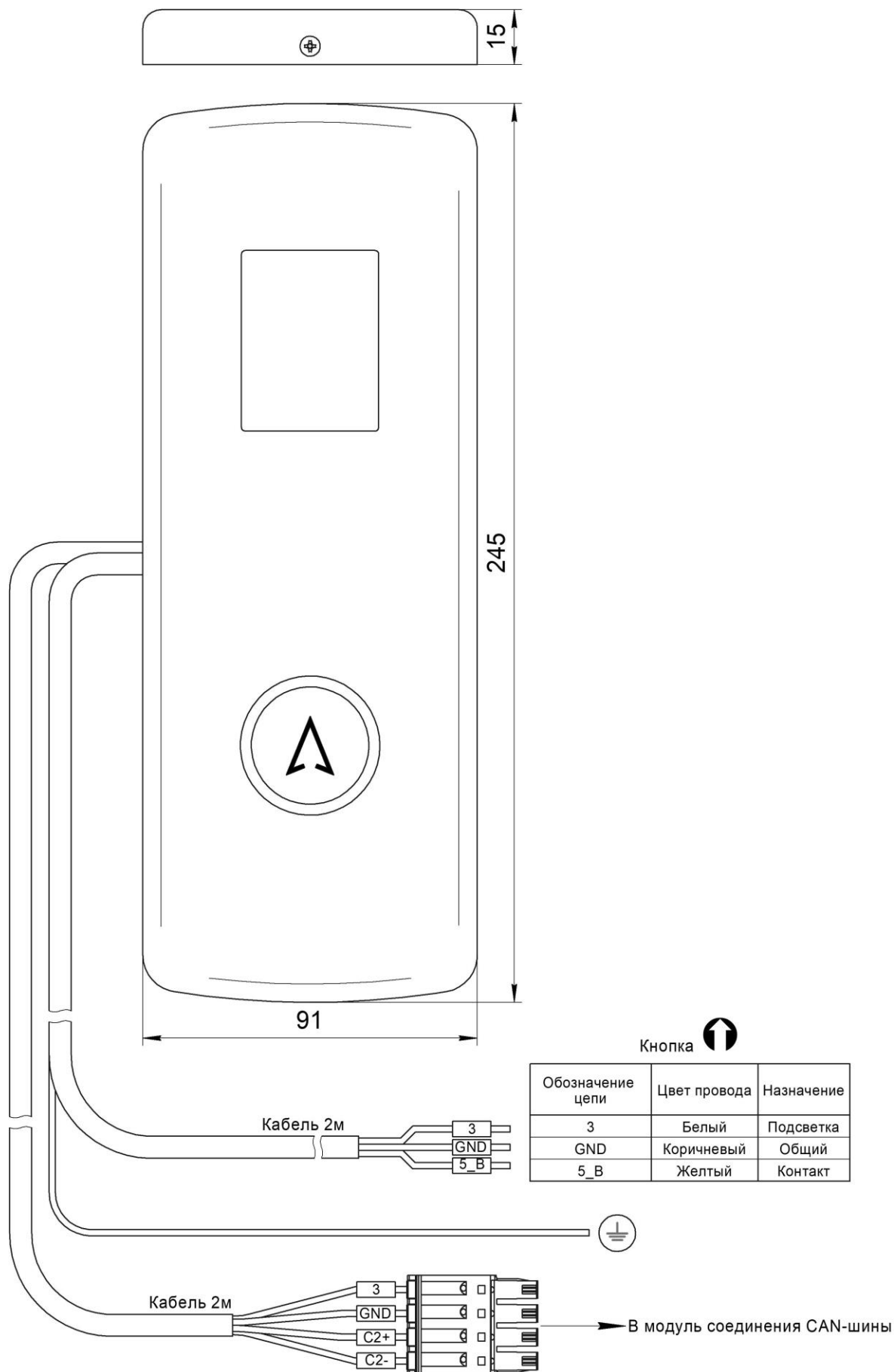
Рис.1 Внешний вид, габаритные и установочные размеры Вызывного поста ЦИРКОН НШЕК.468381.035
